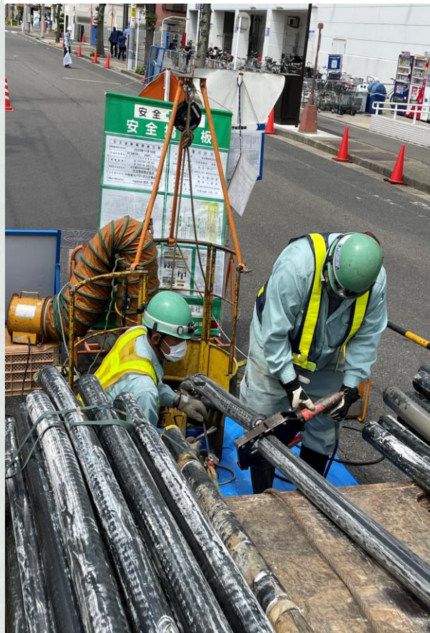
ケーブル切断
